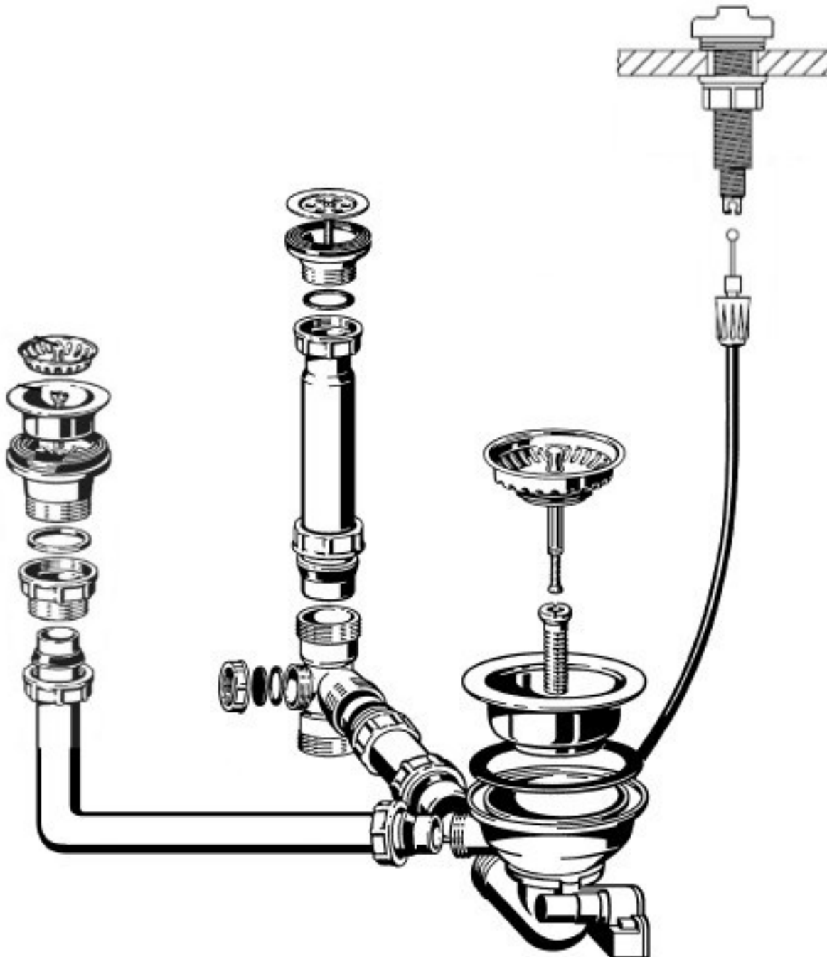
Ablaufgarnitur mit Excenterbetätigung 1 x 3 1/2"
